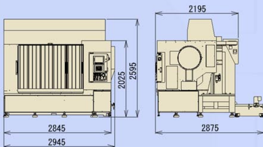
外形寸法図
