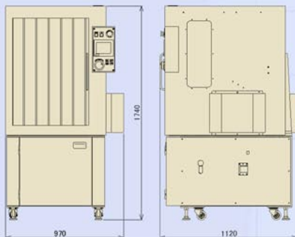
外形寸法図
